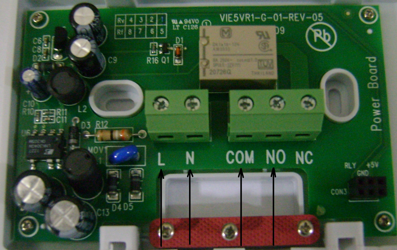
220 VOLT KOMBİ BAĞLANTI UÇLARI
